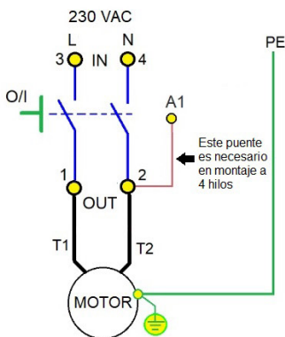
Esquema Eléctrico
