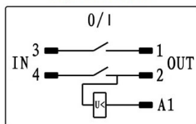
Esquema Eléctrico
