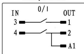
Montaje a 4 hilos
